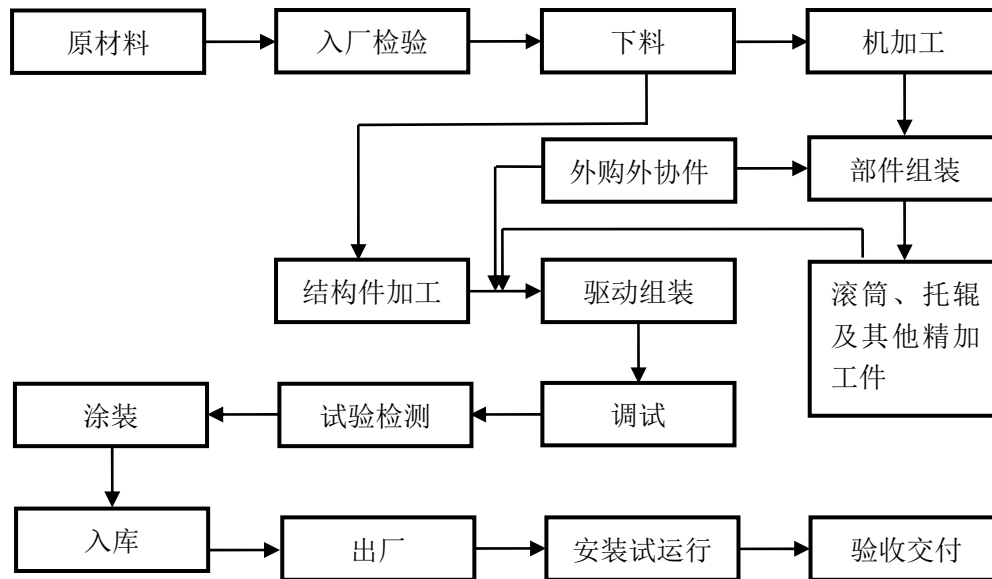
图11-5 输送机械生产工艺流程图
