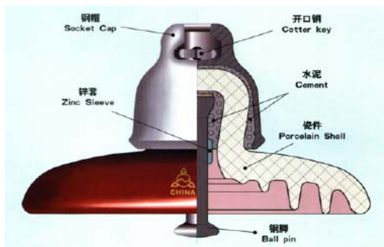
悬式瓷绝缘子结构图
