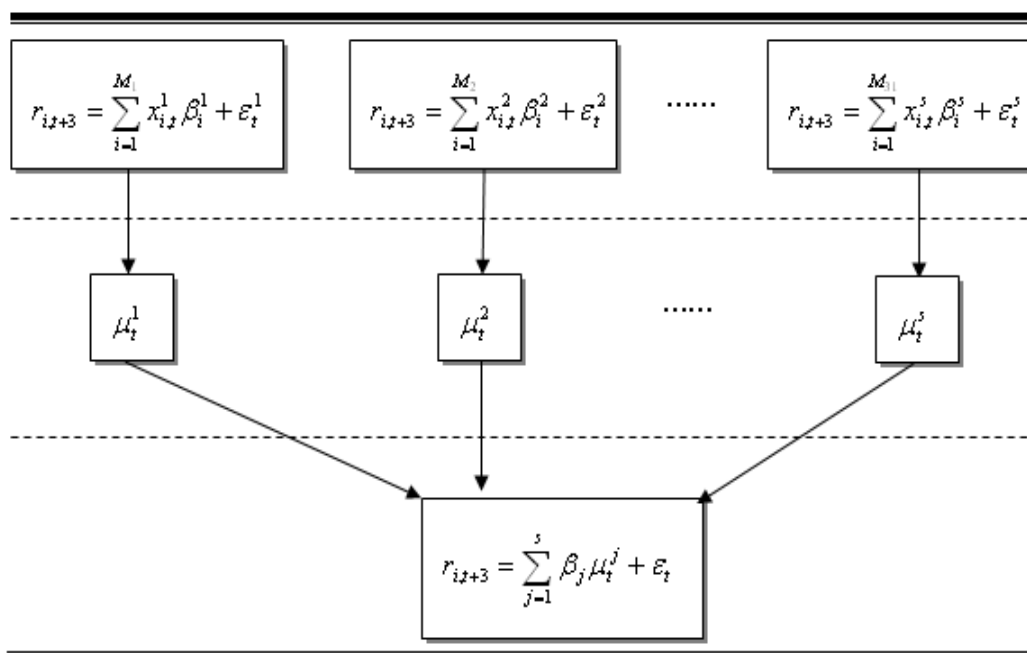
图 2 大成行业收益预测模型构建方法
