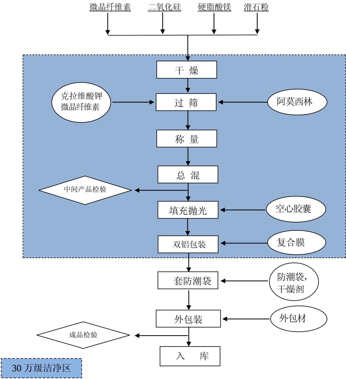
阿莫西林克拉维酸钾胶囊生产工艺流程图
