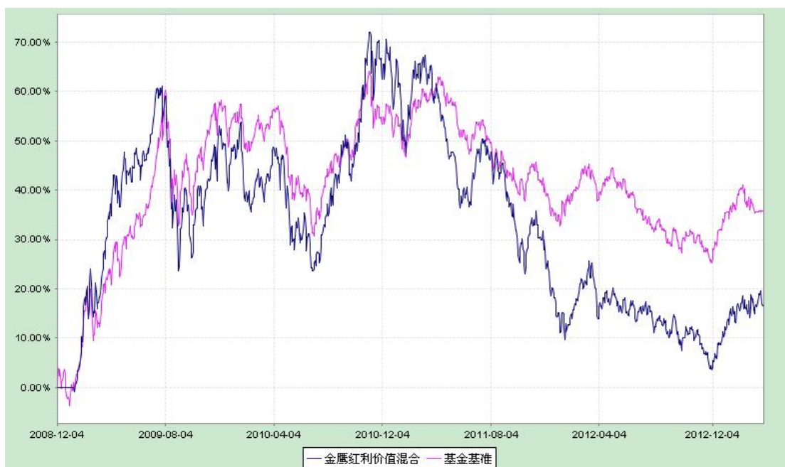
金鹰红利价值混合型基金累计份额净值增长率与同期业绩比较基准收益率的历史走势对比图（2008 年 12 月 4 日至 2013 年 3 月 31 日）
