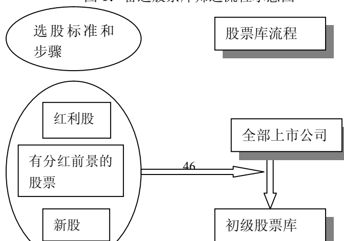
图 1：备选股票库筛选流程示意图
