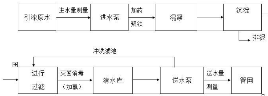
供水业务工艺流程示意图
