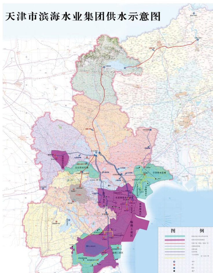
滨海水业供水示意图
