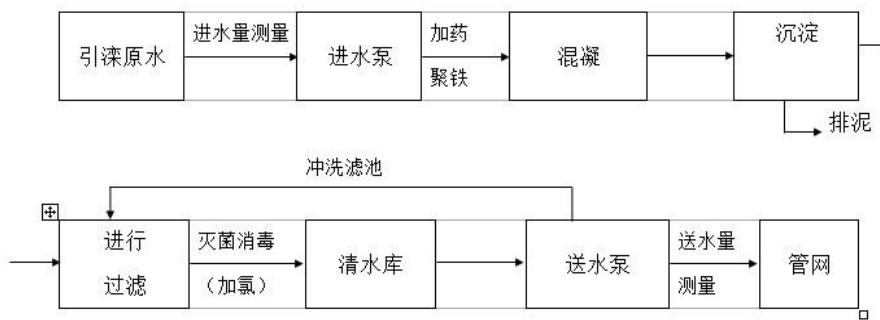
供水业务工艺流程示意图
