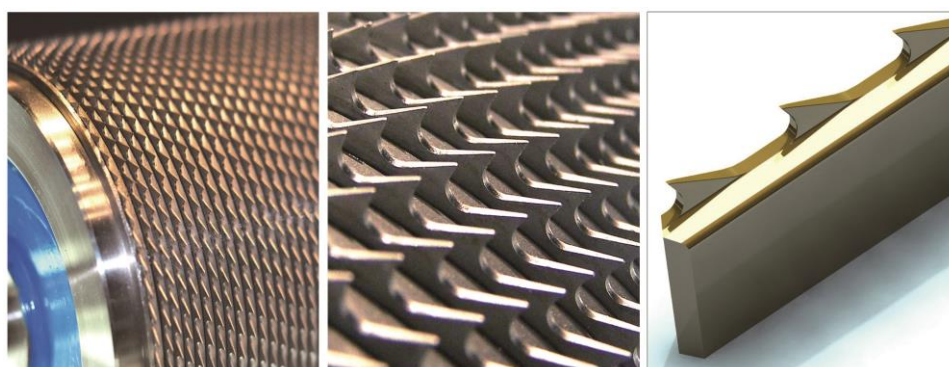
金属针布
