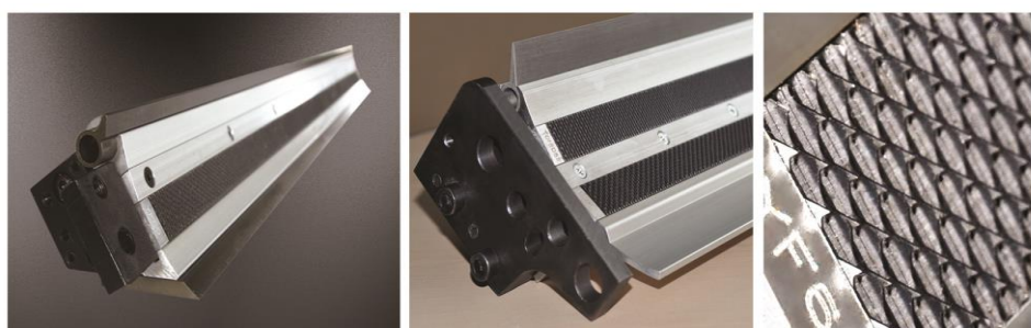
预分梳板
