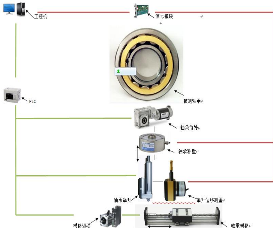
轴承内孔测量产品工作原理示意图
