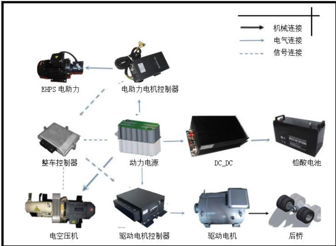
福建万润纯电动动力系统连线图
