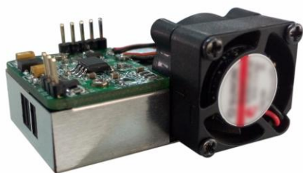
图2 激光PM2.5粉尘传感器
