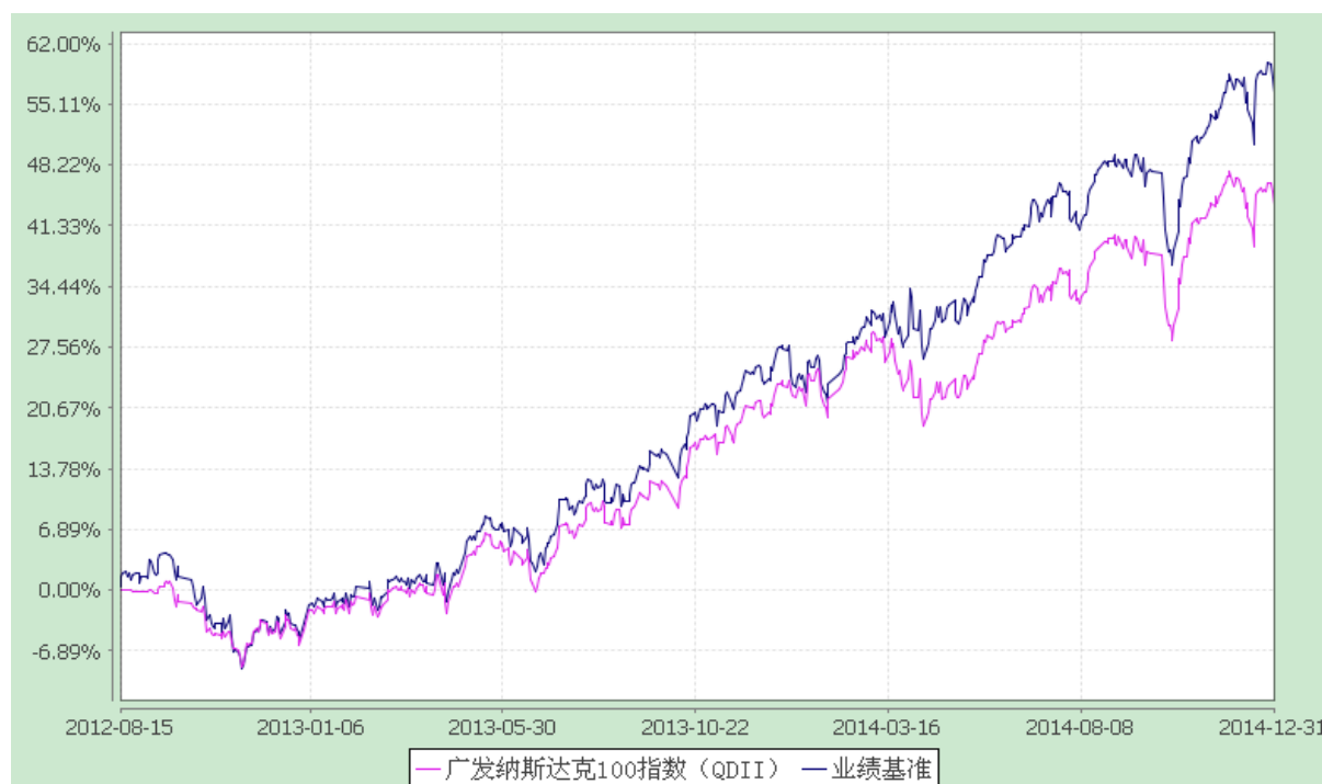
广发纳斯达克 100 指数证券投资基金 份额累计净值增长率与业绩比较基准收益率历史走势对比图 (2012 年 8 月 15 日至 2014 年 12 月 31 日)
