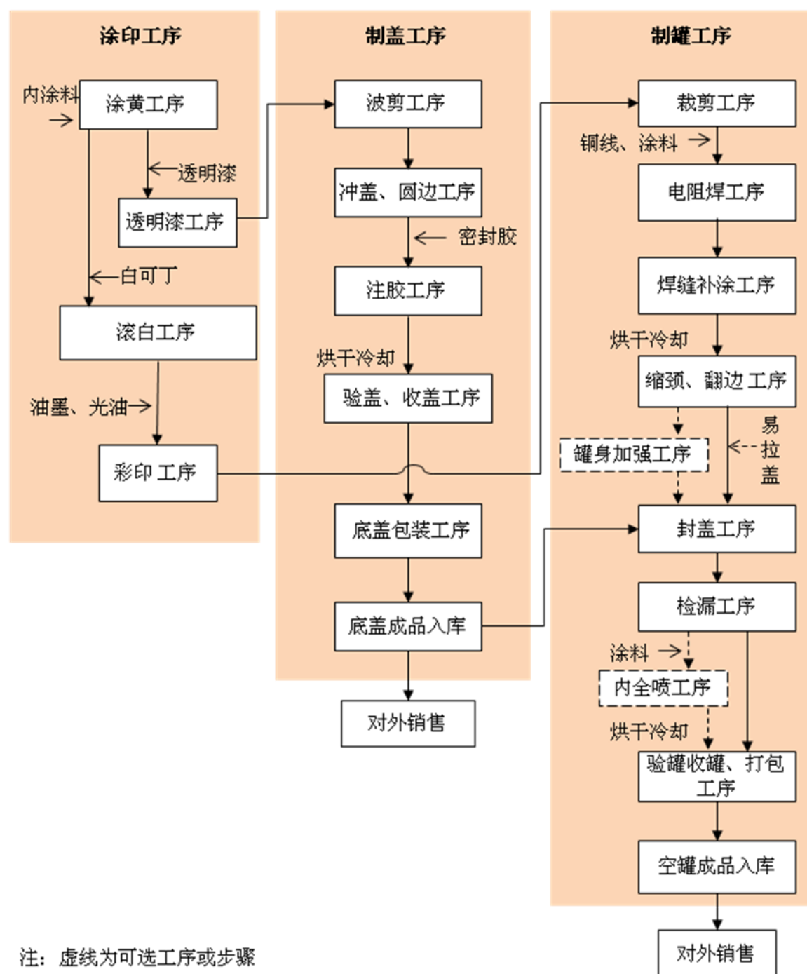
马口铁三片罐生产工艺流程图
