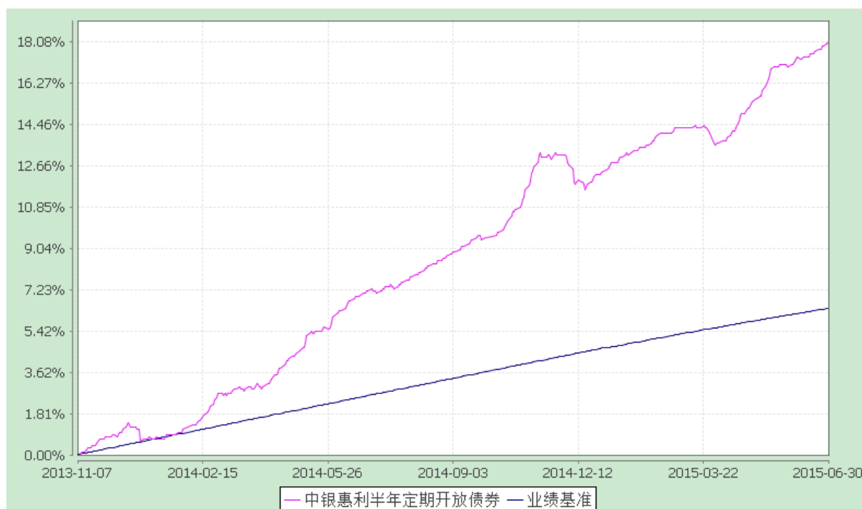
中银惠利纯债半年定期开放债券型证券投资基金 份额累计净值增长率与业绩比较基准收益率历史走势对比图 （2013 年 11 月 7 日至 2015 年 6 月 30 日）
