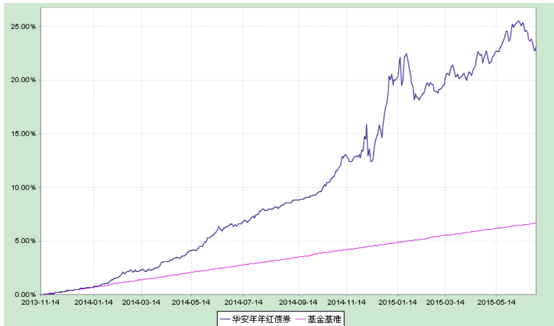
华安年年红定期开放债券型证券投资基金 累计净值增长率与业绩比较基准收益率历史走势对比图 (2013 年 11 月 14 日至 2015 年 6 月 30 日)
