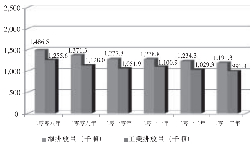
二零零八年至二零一三年 中國的整體及工業顆粒物排放
