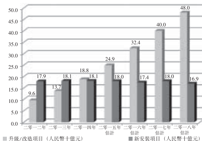
中國新安裝項目及升級／改造項目的除塵器銷售額
