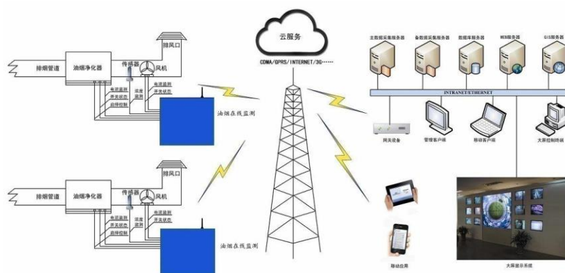
图1 油烟在线监测系统
