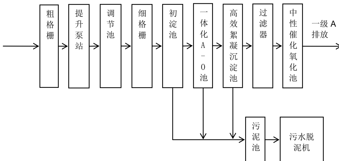
(2) 工业废水处理工艺流程图
