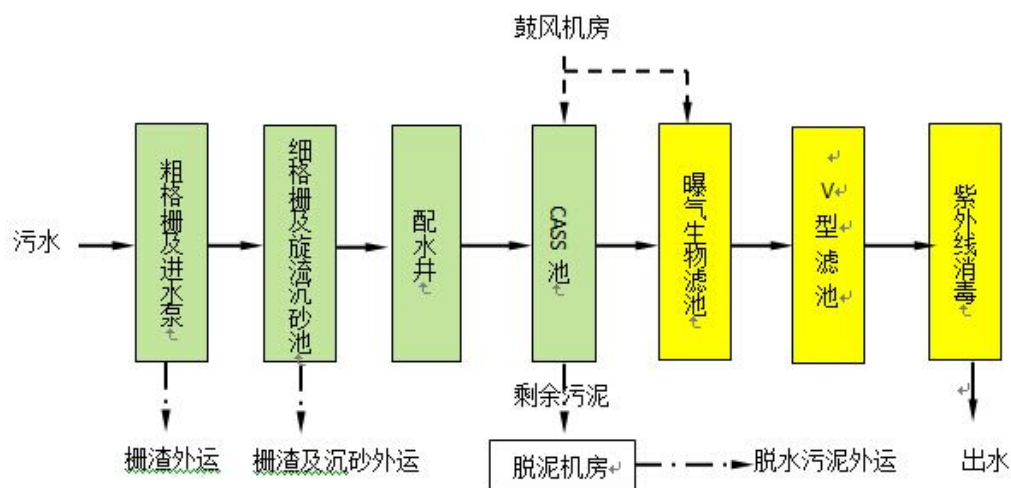
图 1—工艺流程图
