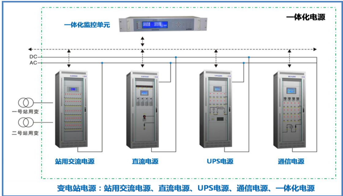
附：站用电电源系统图
