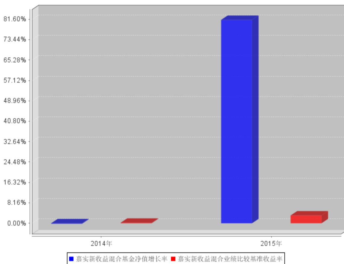
嘉实新收益混合自基金合同生效以来基金每年净值增长率及其与同期业绩比较基准收益率的对比图
