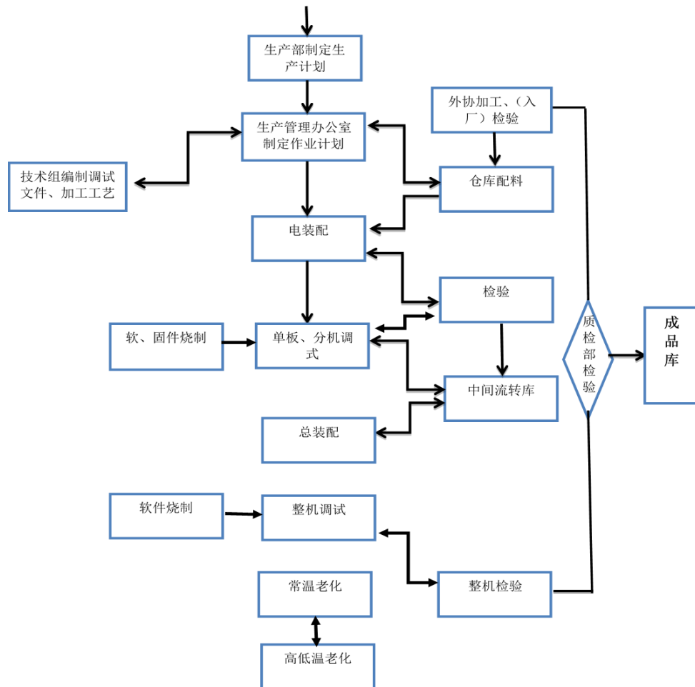
生产工艺流程图
