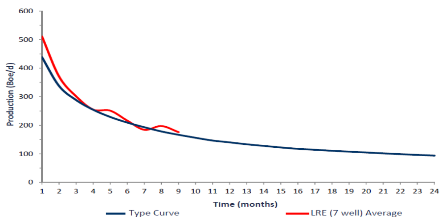
D、Deep Basin—Wapiti区（Kakwa）区域单井的月产量标准曲线图
