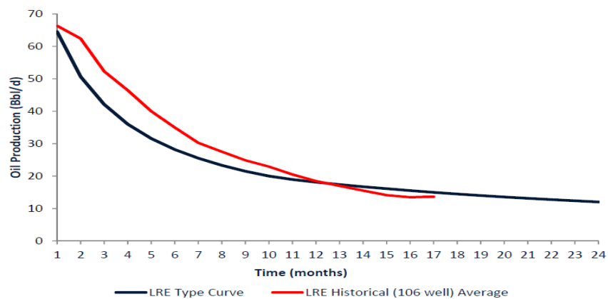
C、Deep Basin区域—Edson区 (Pine Creek) 单井的月产量标准曲线图
