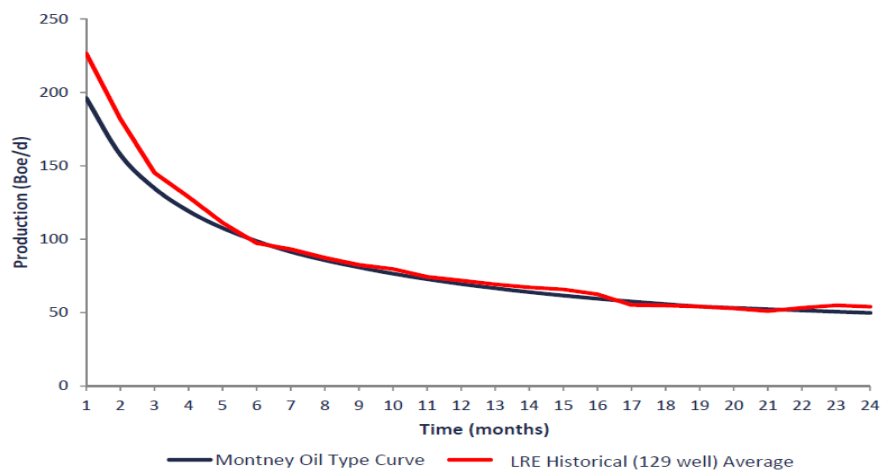
B、Redwater区域单井的月产量标准曲线图
