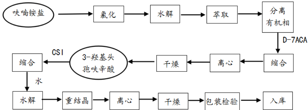
(6) 头孢呋辛酸生产流程图
