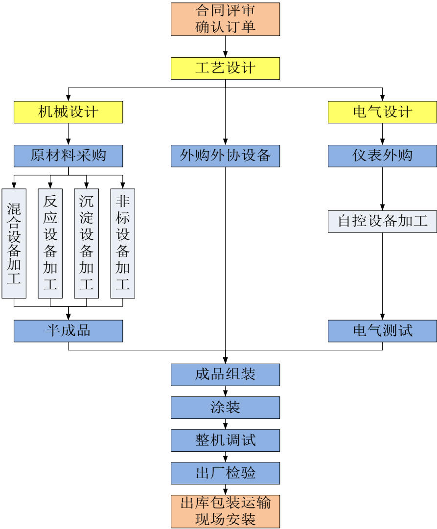
（2）核心自产设备生产工艺流程图
