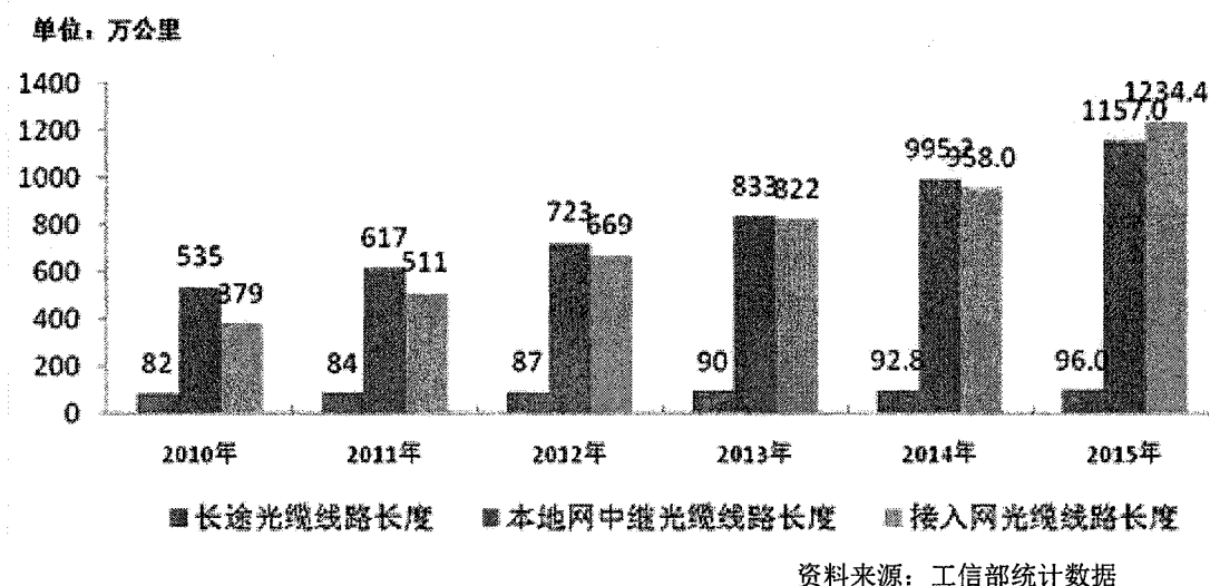
图5-19 2010-2015 年各种光缆线路长度对比情况
