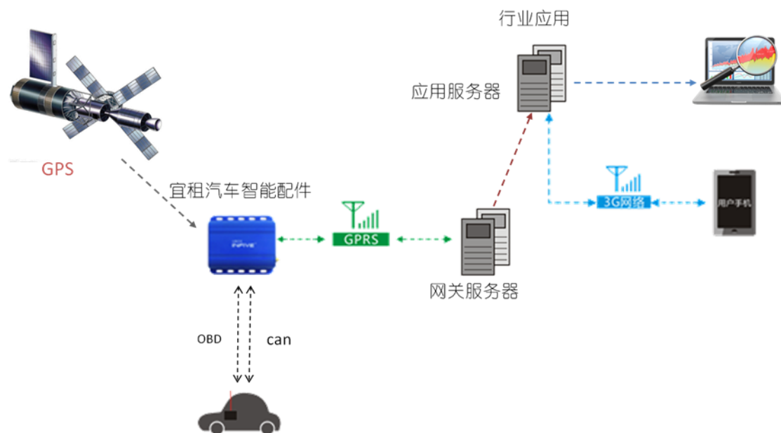
宜租车联网架构原理图
