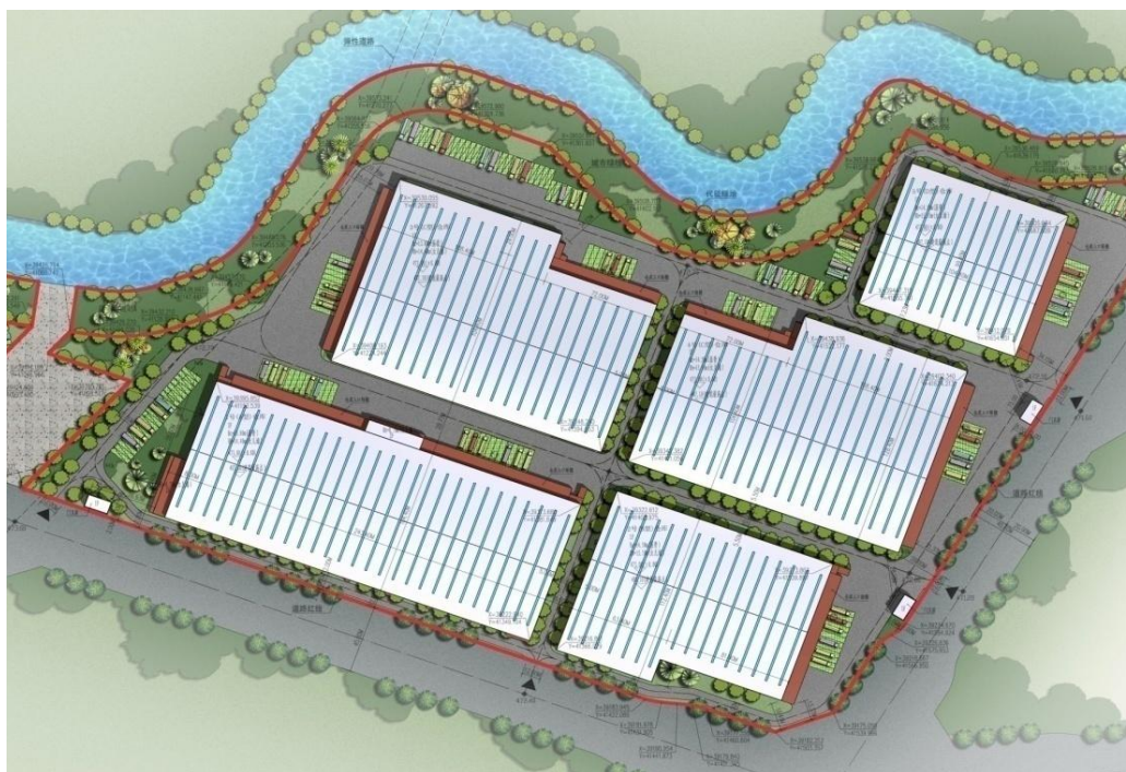
图13-1 本项目建设总平面图
