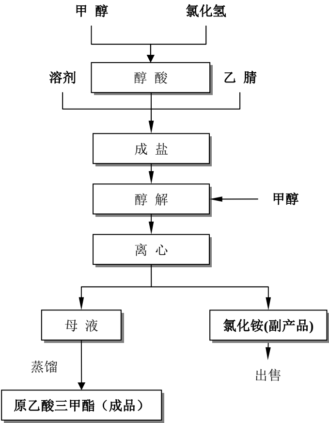
图 6-12：原乙酸三甲酯的生产工艺流程
