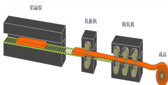
铝压延业务生产流程
