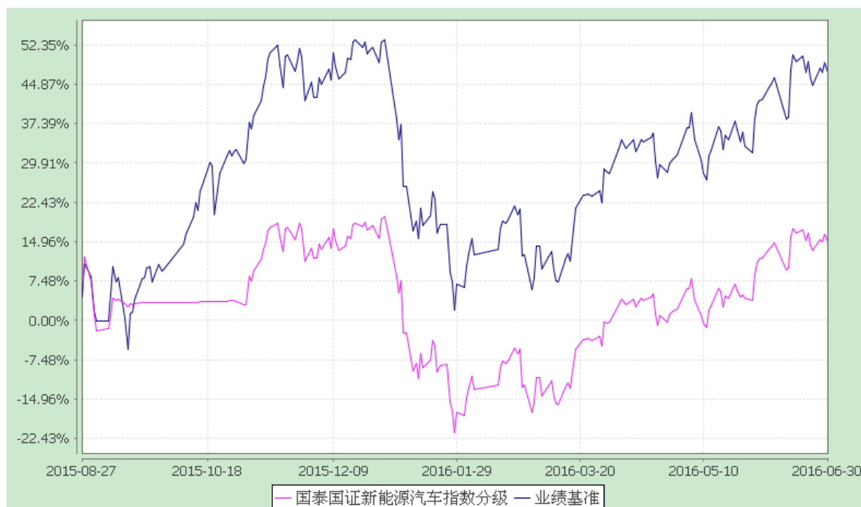
自基金转型以来份额累计净值增长率与业绩比较基准收益率历史走势对比图 (2015 年 8 月 27 日至 2016 年 6 月 30 日)
