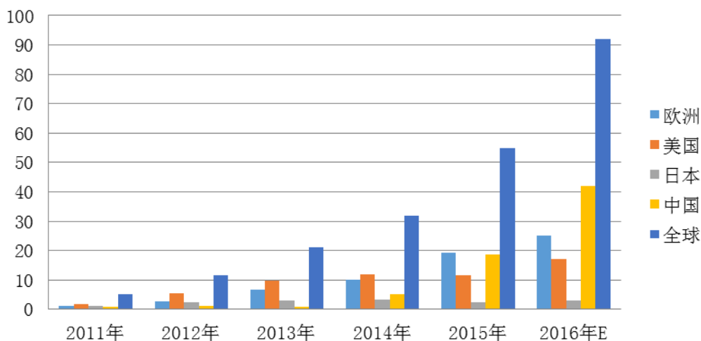
全球主要国家新能源电动汽车销量情况（万辆）
