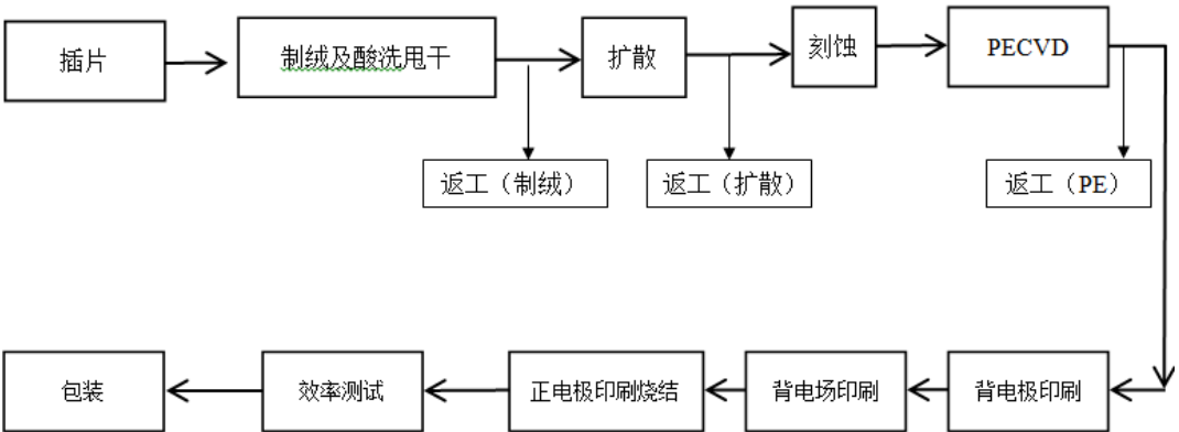
多晶硅太阳能电池生产工艺流程
