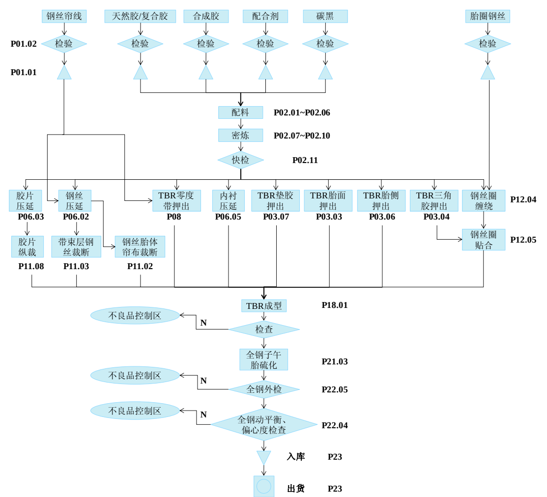
(2) 全钢子午胎生产工艺流程
