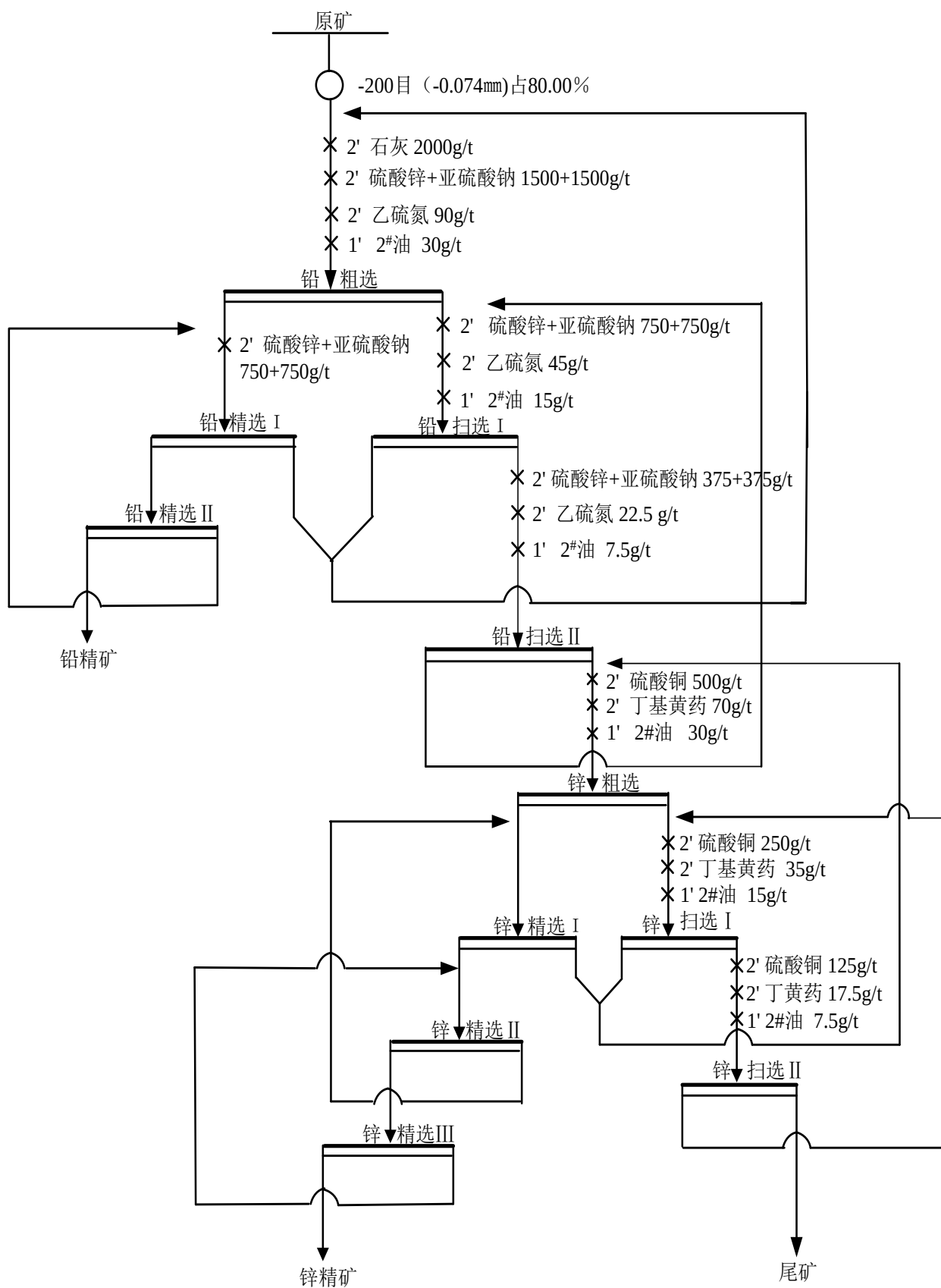
银铅锌矿石选矿工艺流程图
