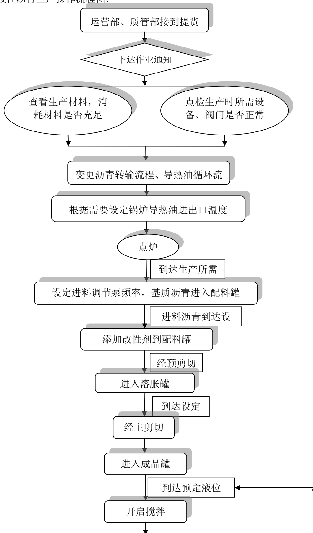
改性沥青生产操作流程图：
