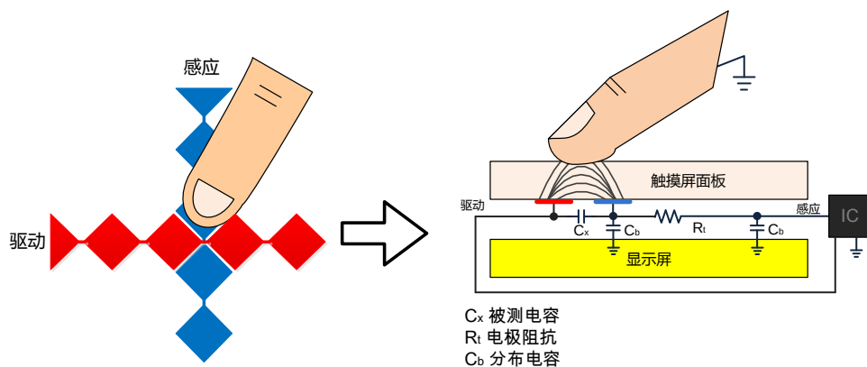
图 2 互容电容检测原理
