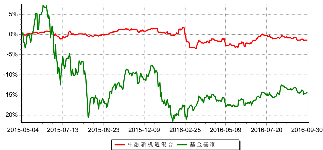
中融新机遇灵活配置混合型证券投资基金 份额累计净值增长率与同期业绩比较基准收益率历史走势对比图 (2015年05月04日至2016年09月30日)
