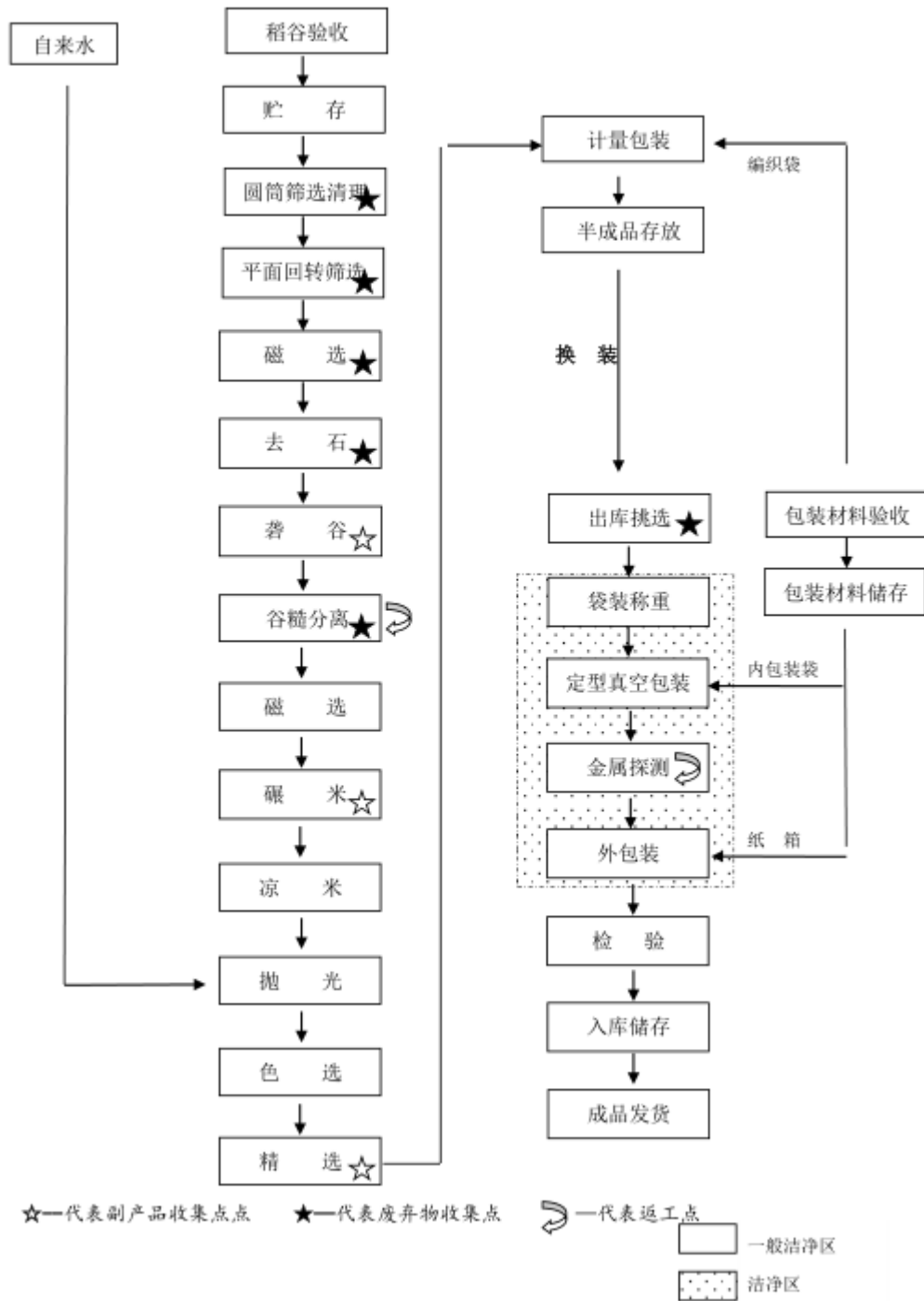
大米生产工艺流程图
