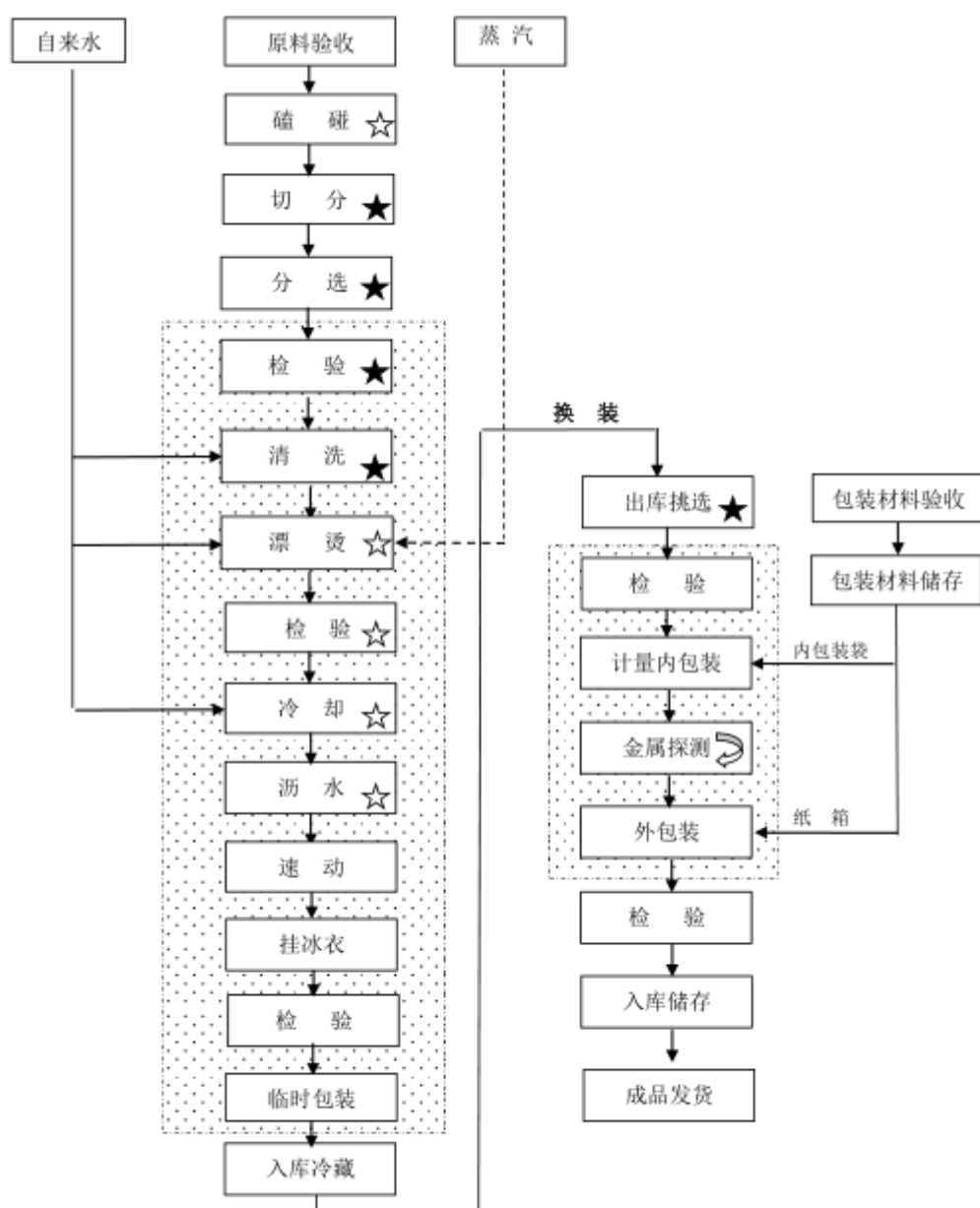
IQF 西兰花生产工艺流程图
