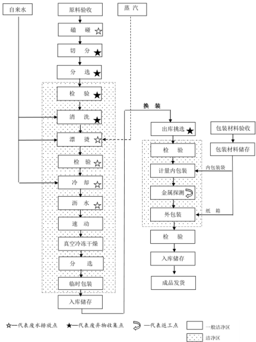
FD 西兰花生产工艺流程图
