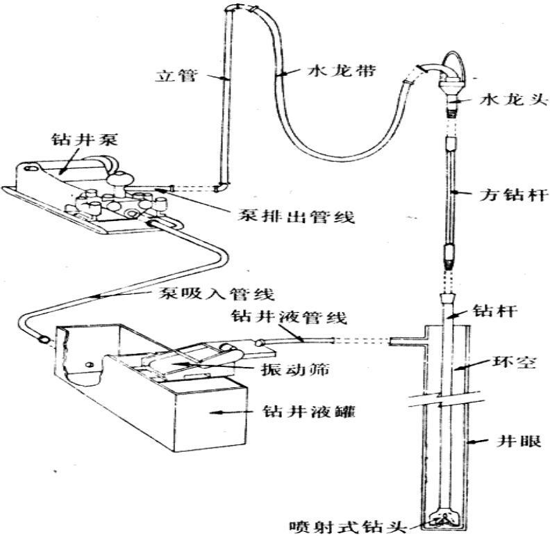
公司钻井液循环系统运行模式
