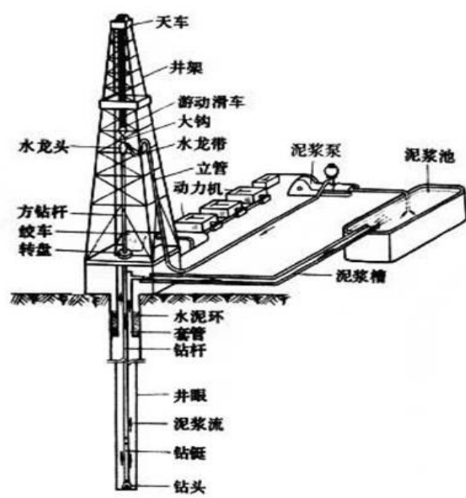
钻机示意图
