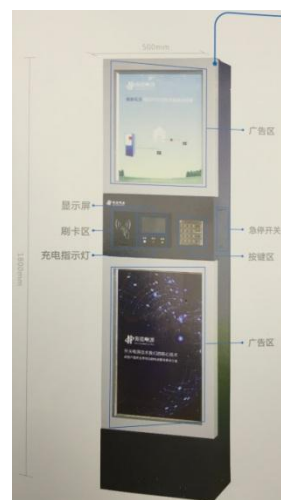
图 7 媒体广告型交流充电桩
