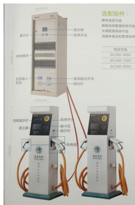
图 4：分体式直流充电桩
