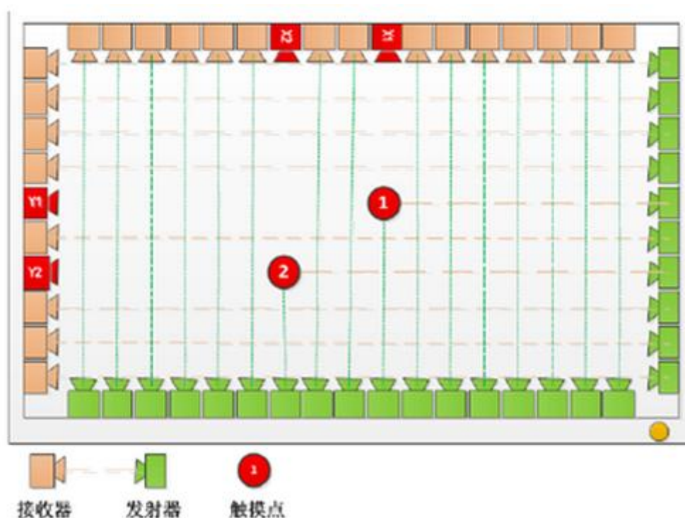
红外线式触摸屏工作原理图
