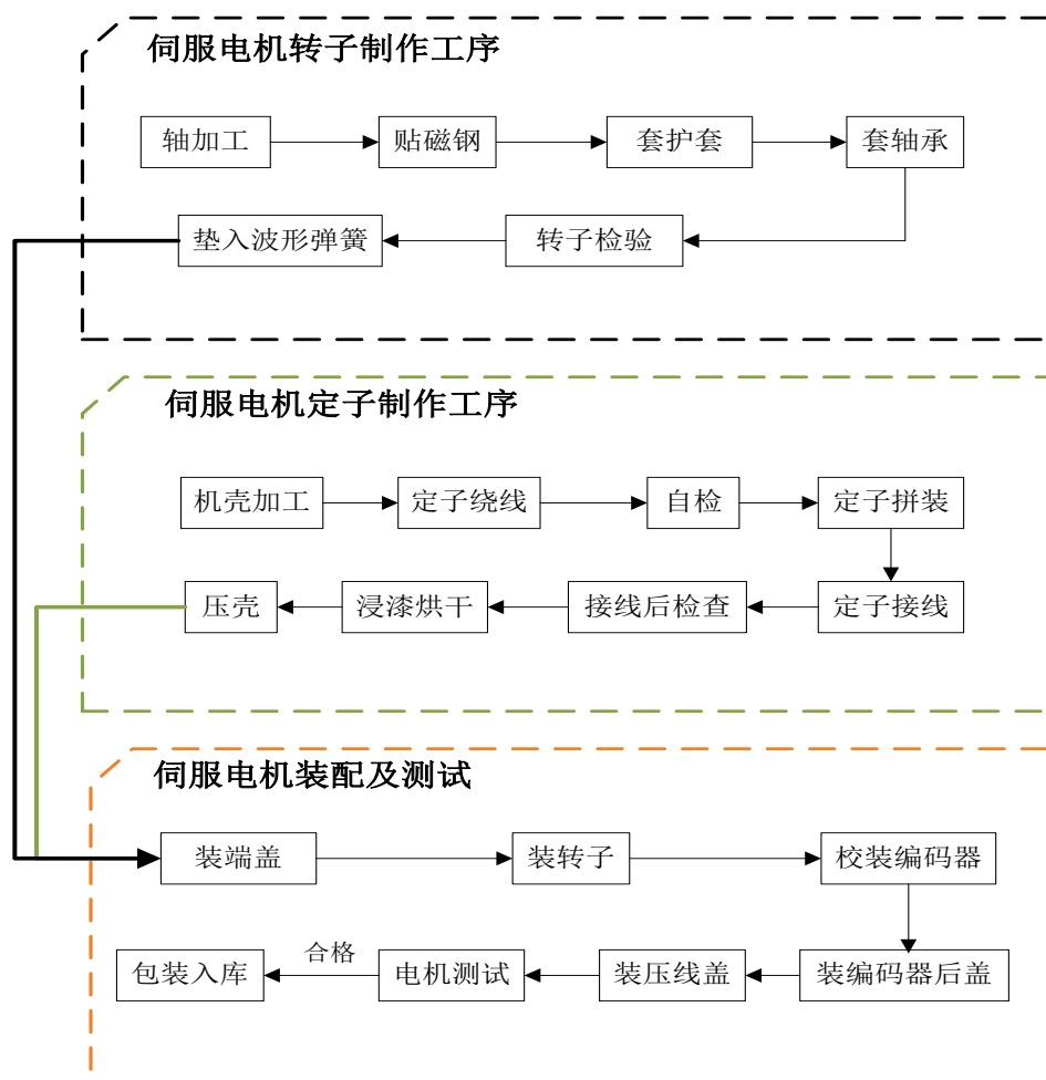
伺服电机生产流程图
