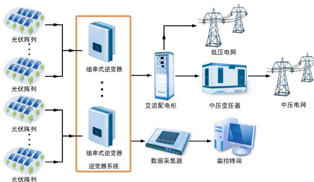
组串式逆变器发电示意图
