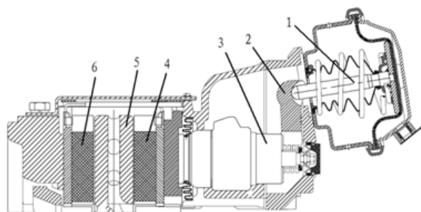
1、气室顶杆 2、压力臂 3、转动组件 4、内摩擦块 5、制动盘 6、外摩擦块 1、 Air chamber push rod 2、 Lever 3、 Adjuster 4、 Inner pad 5、 Brake disc 6、 Outer pad
