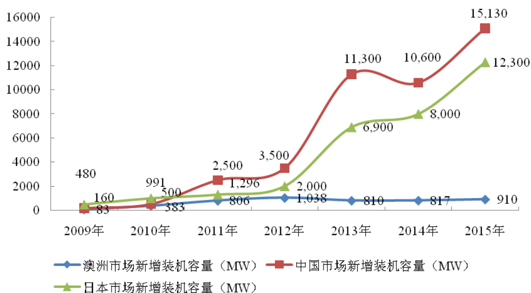
2009 年-2015 年中国、日本、澳洲市场新增装机容量变化图
