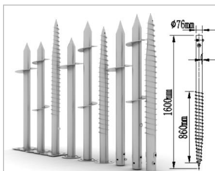
钢制地桩
