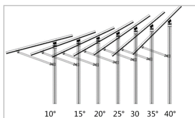
预装三角结构
