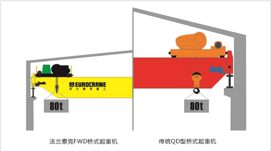
公司设计的 80 吨的起重机与传统设计的起重机对比图
