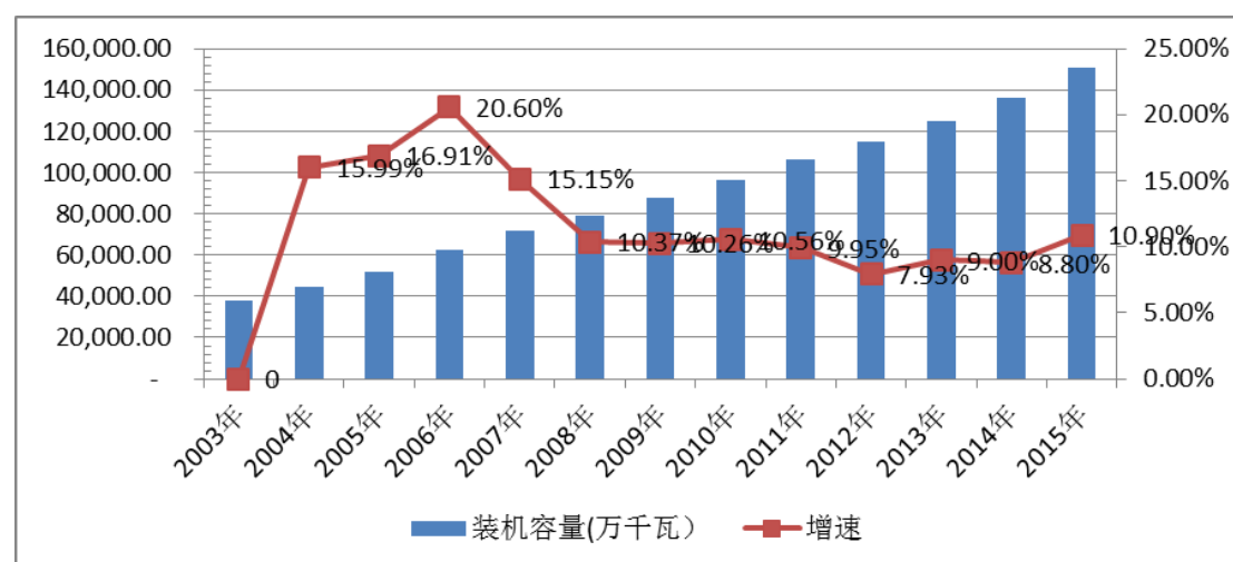
2003 年-2015 年我国装机容量
