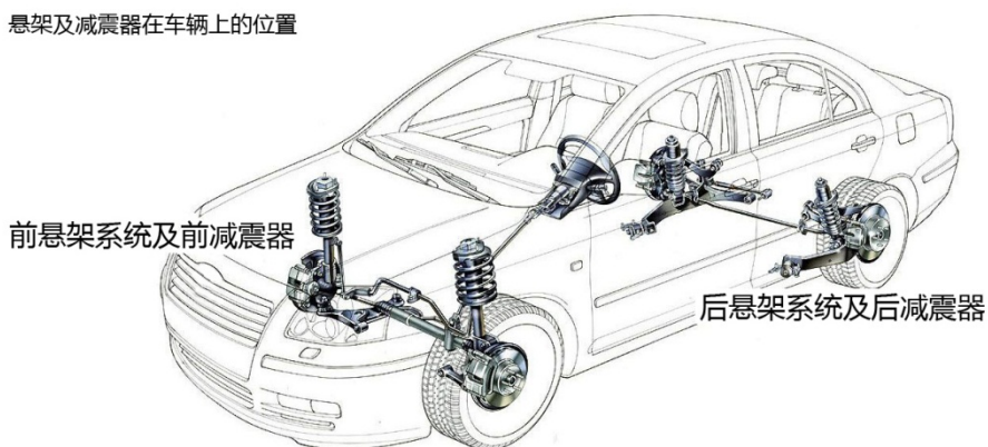
悬架及减震器在车辆上的位置
