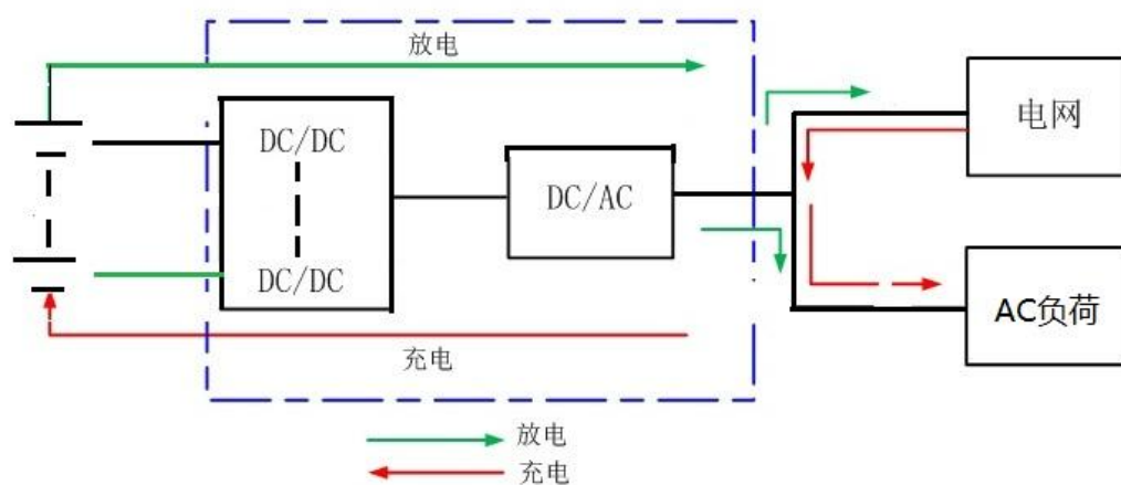
(2) 能量回馈型电源系统
