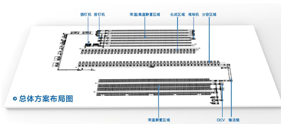
② 全自动化系统结构图
