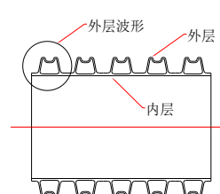
图：发行人优化设计波纹管结构图
