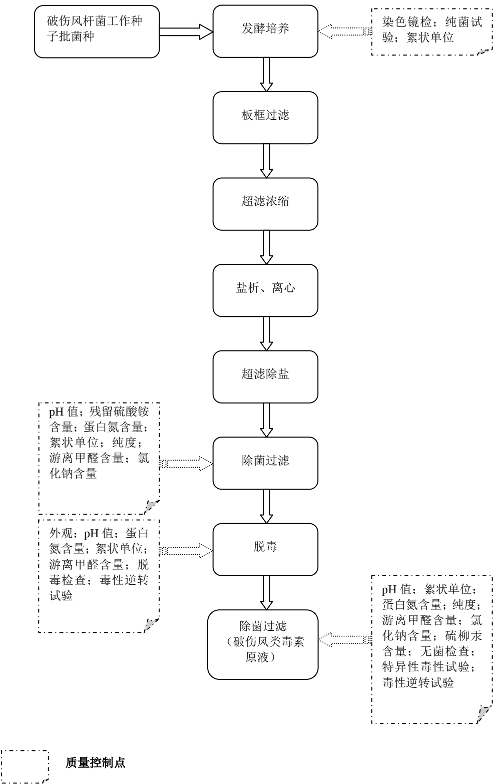
(4) 破伤风类毒素原液生产工艺流程图
