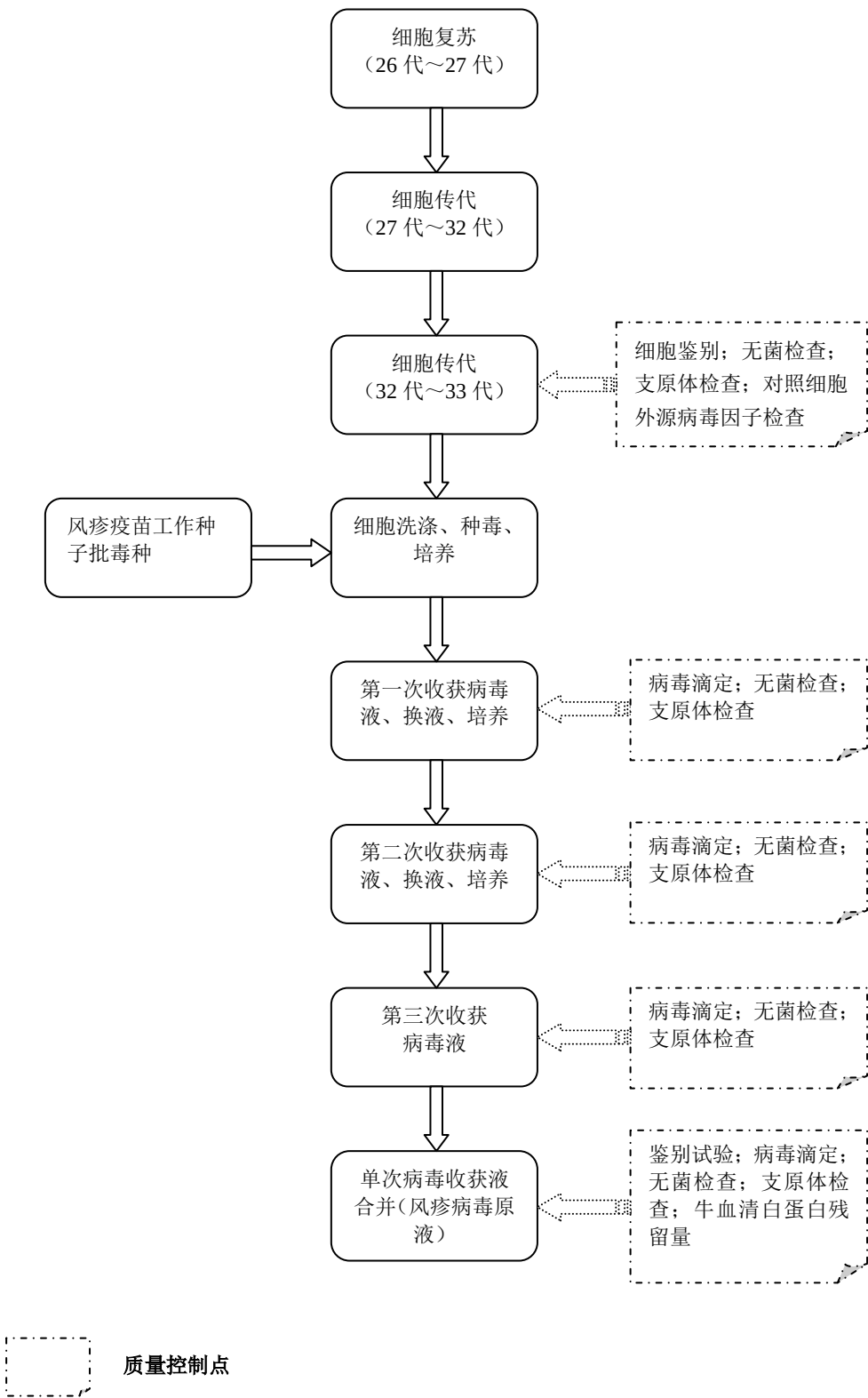
(2) 风疹病毒原液生产工艺流程图
