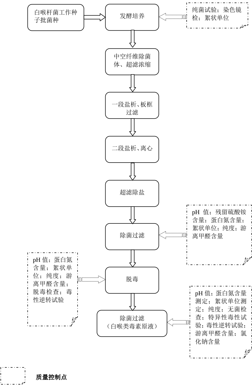
(3) 白喉类毒素原液生产工艺流程图
