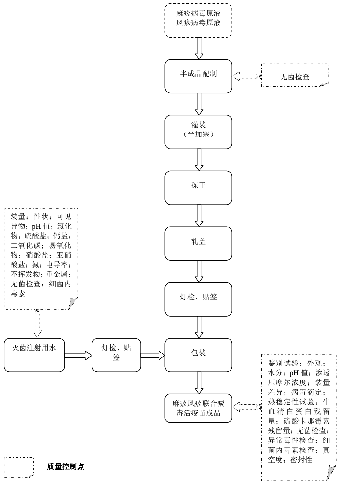
(3) 麻风二联苗分包装生产工艺流程图
